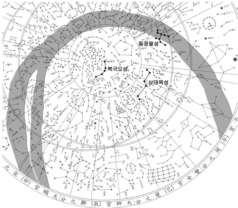
〈그림 5〉 조선시대 天象列次分野之圖의 은하수와 東井八星 (회색 띠는 은하수)
